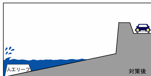
構造物設置による越波対策の例
